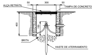
CORTE AA'
